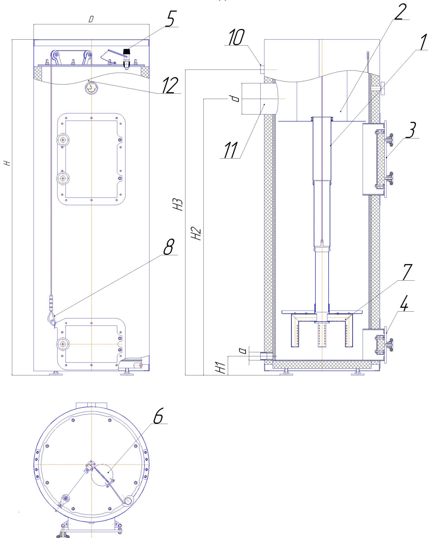
Рис. 1. Габаритные и присоединительные размеры версии "COMFORT"
