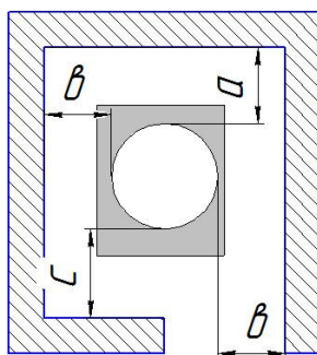
Рис.5 Схема расположения котла
