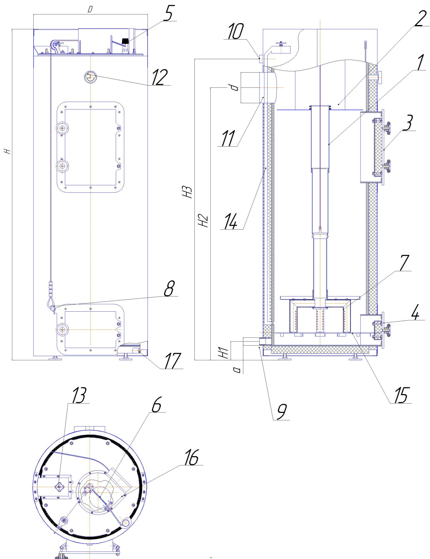
Рис. 2. Габаритные и присоединительные размеры универсальной версии "COMFORT G"
